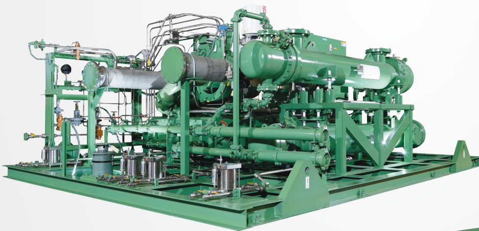
TURBO-GAS 6040
